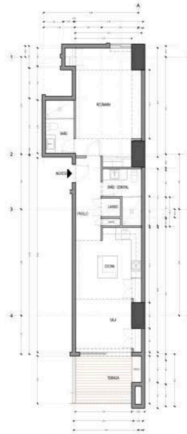
PLANTA ARQUITECTONICA UNIDAD TPO-09
