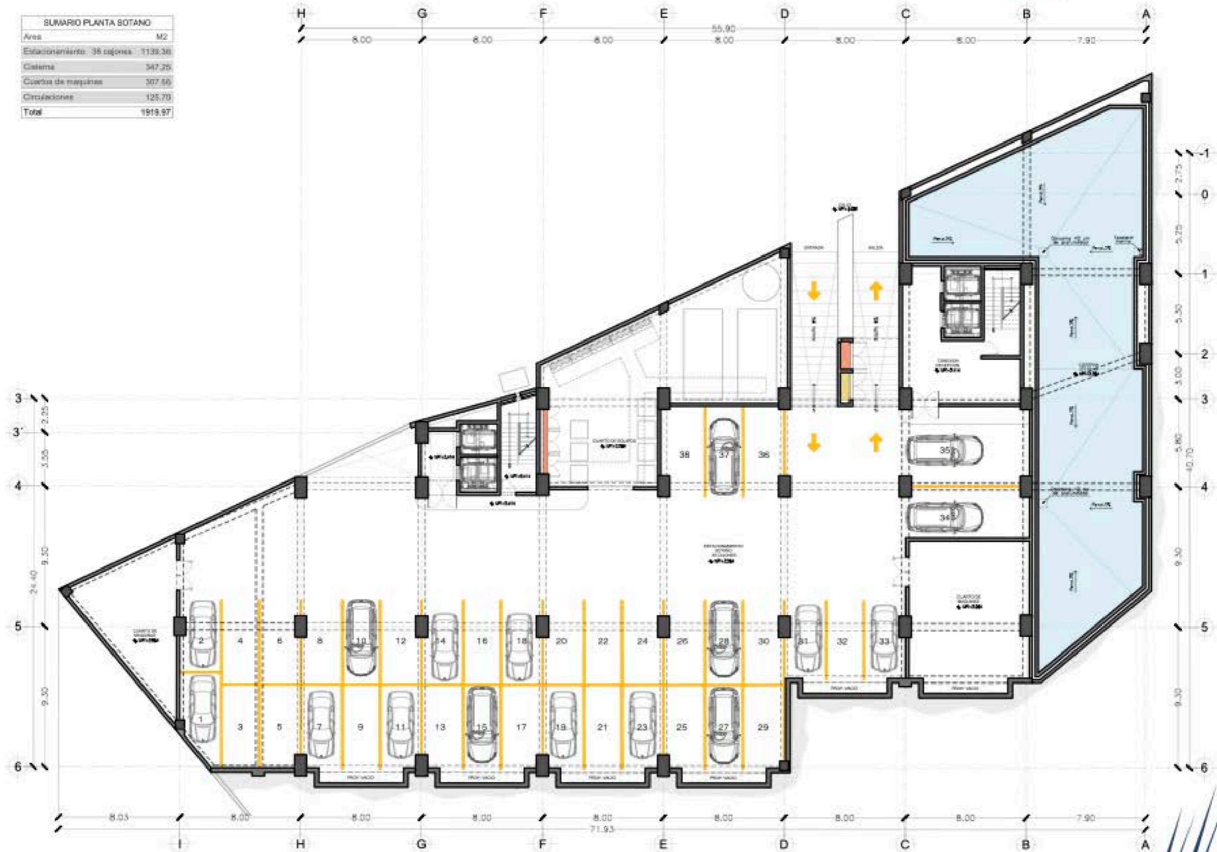
PLANTA ARQUITECTONICA PLANTA SOTANO ESTACIONAMIENTO
